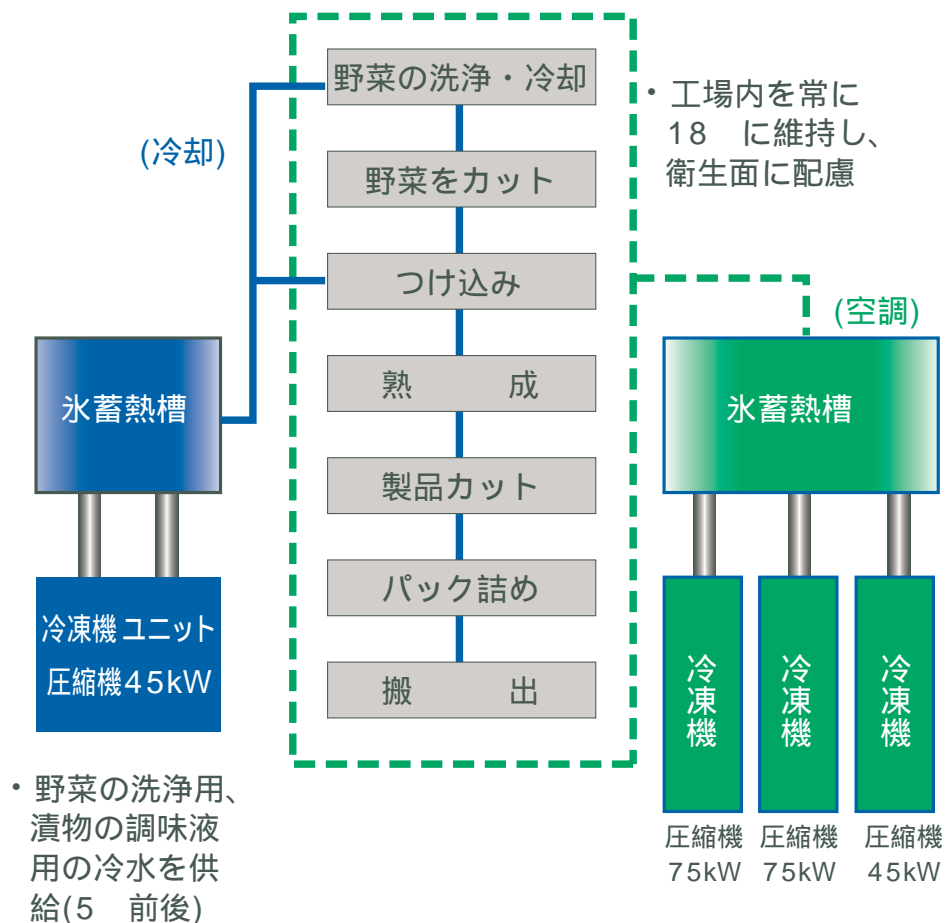
システム図
